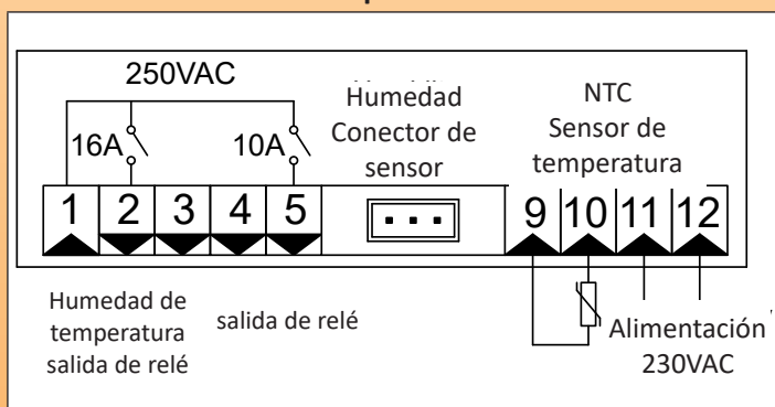
Diagrama de cableado del controlador de humedad y temperatura
